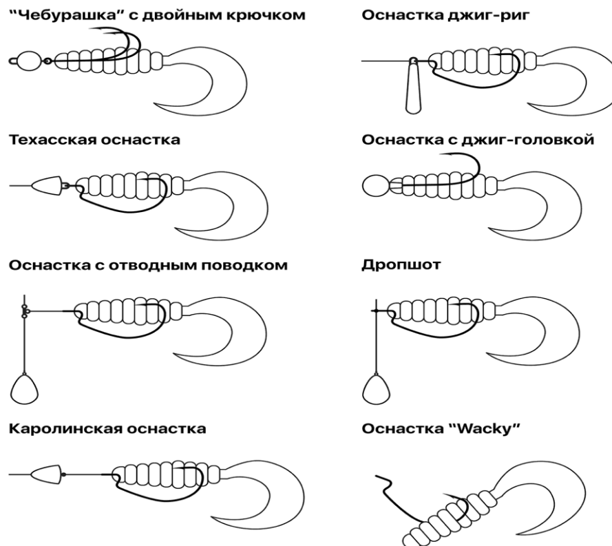
Рис. 2. Оснастки
